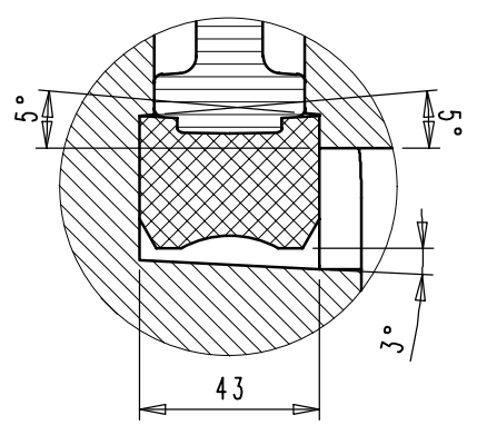
DETTAGLIO g SCALA 1:2
